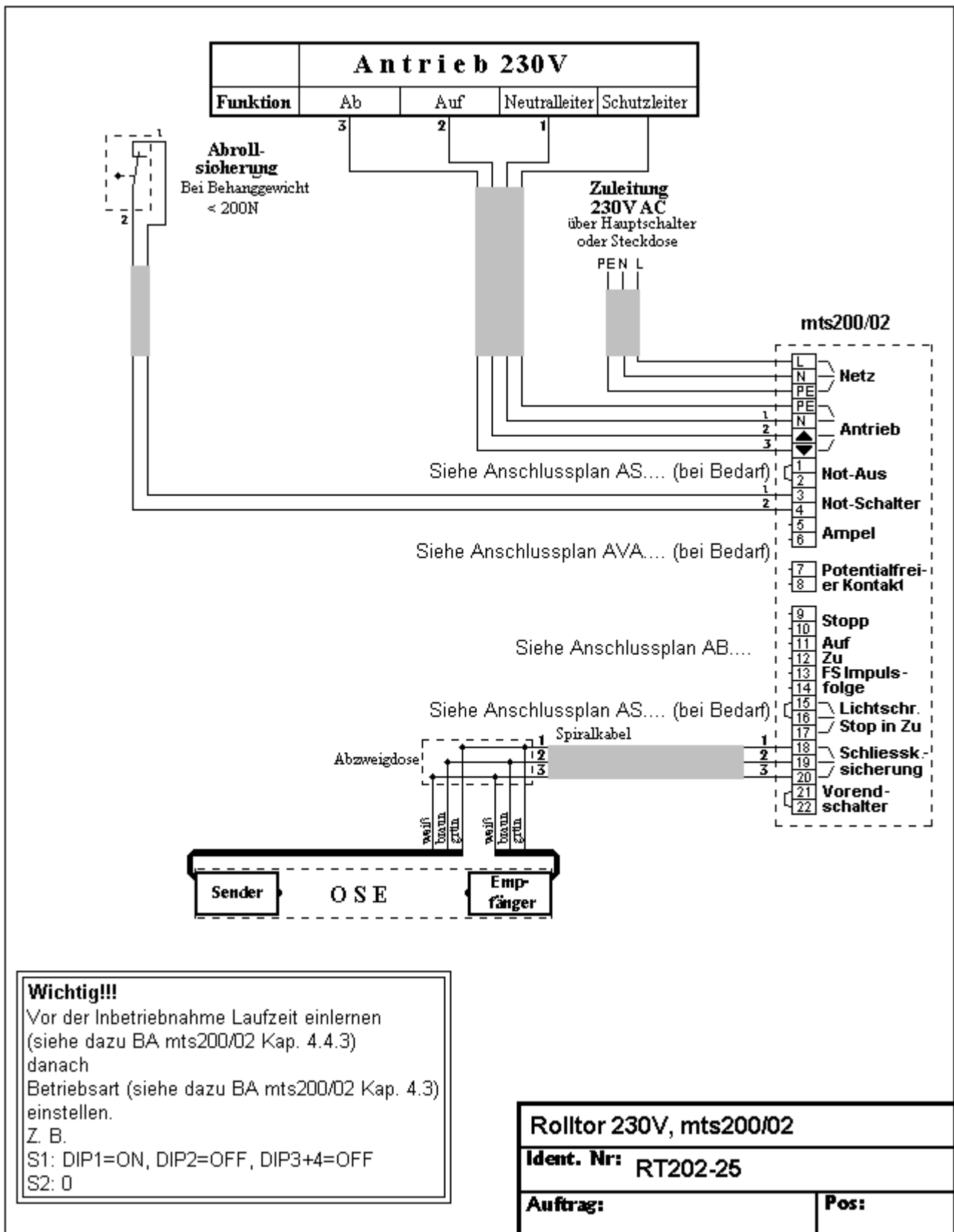
Abb. 10: Anschlussplan mts200/02
