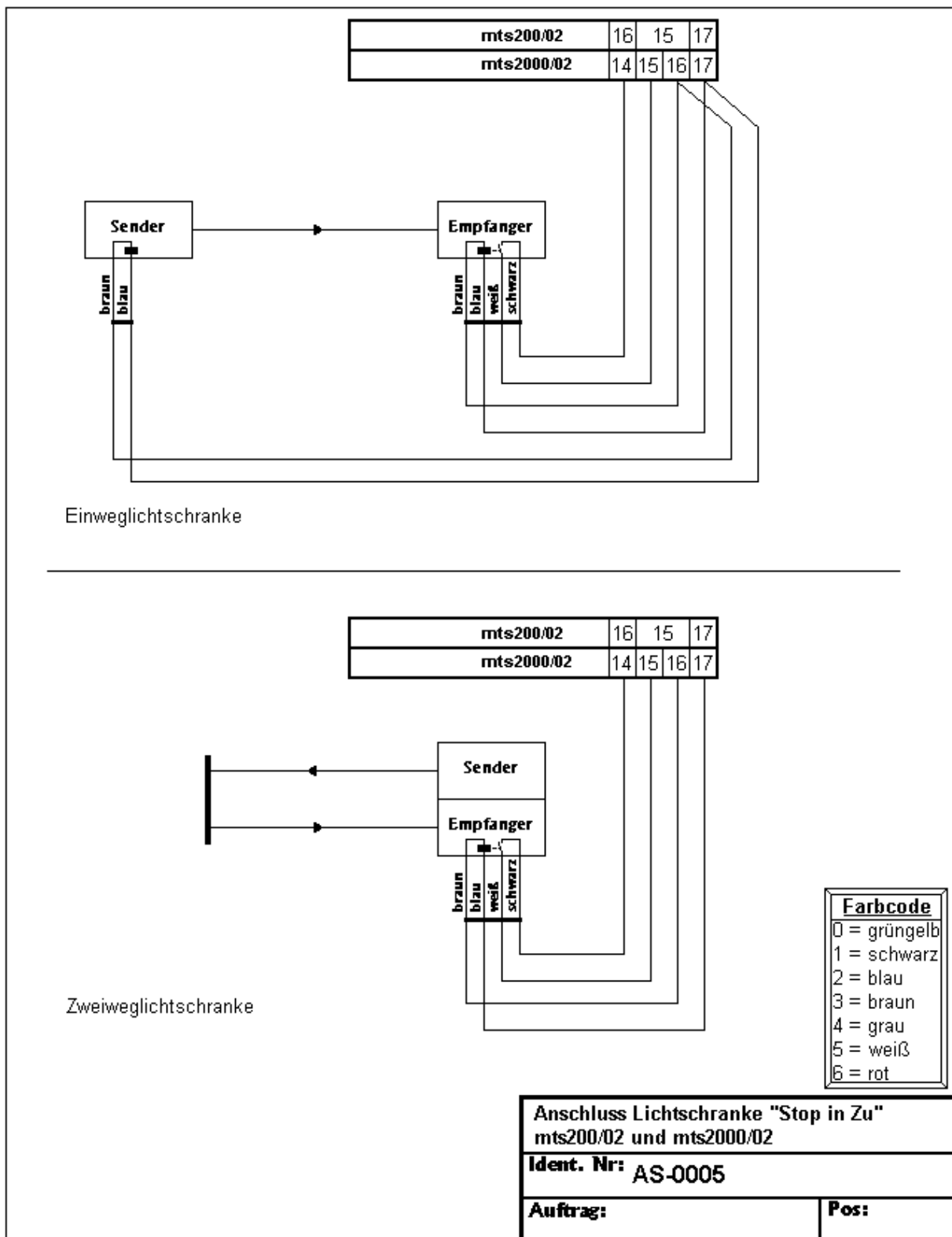
Abb. 12: Lichtschranke
