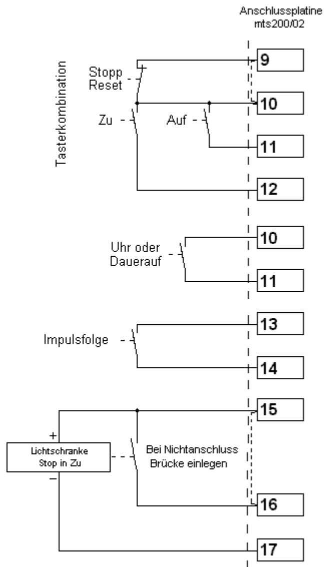
Abb. 7: Anschluss Klemmen 9 – 17 (24VDC)
