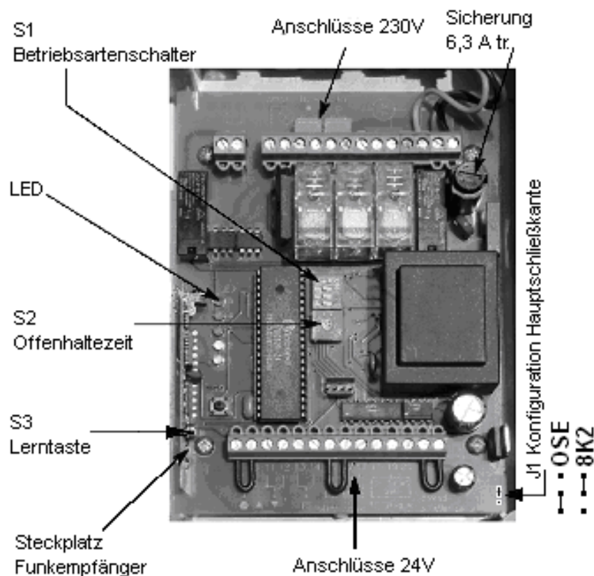
Abb. 1: Steuerplatine
