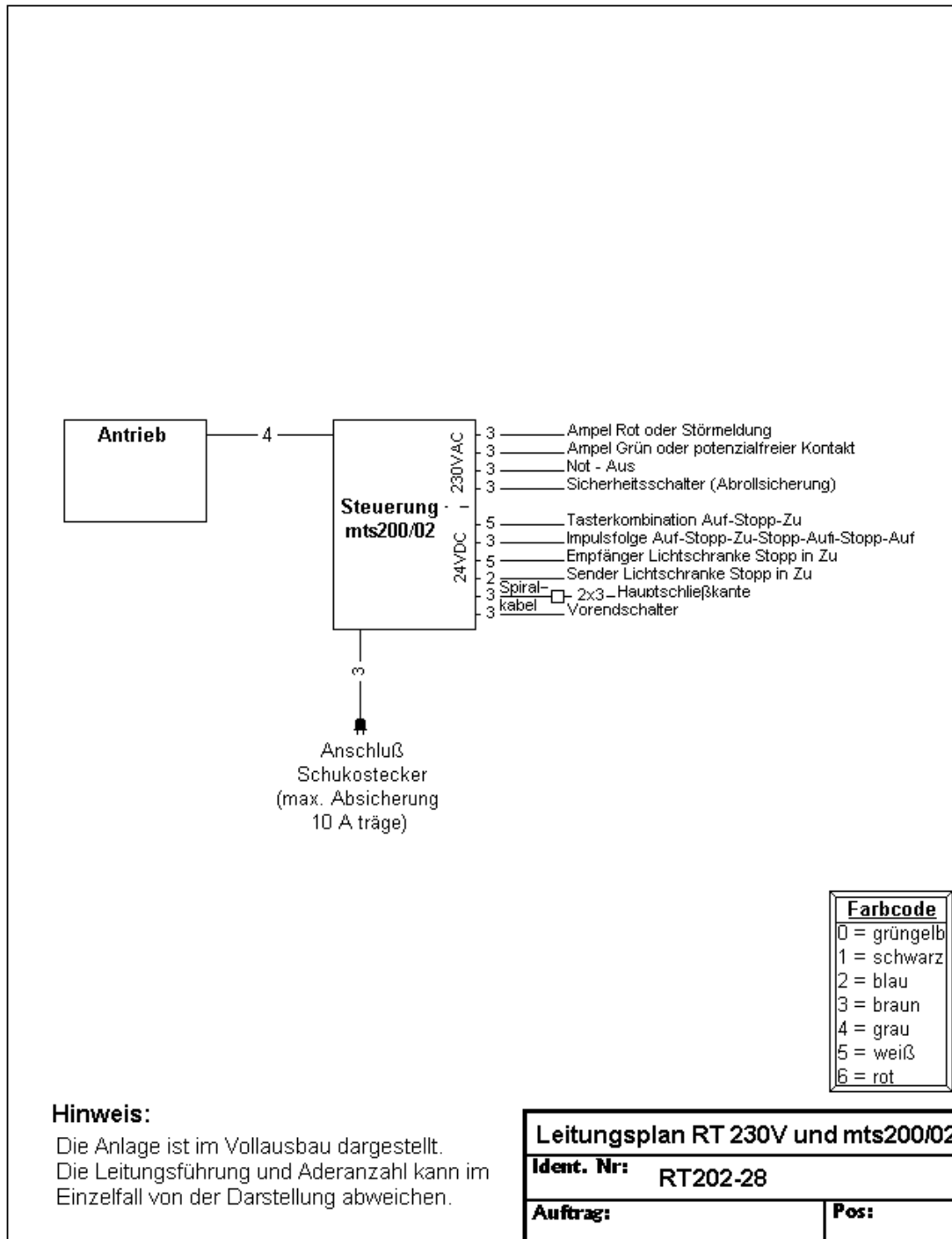
Abb. 9: Leitungsplan
