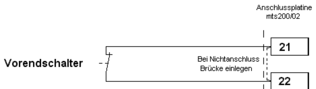
Abb. 8: Anschluss Klemmen 18 – 22 (24VDC)
