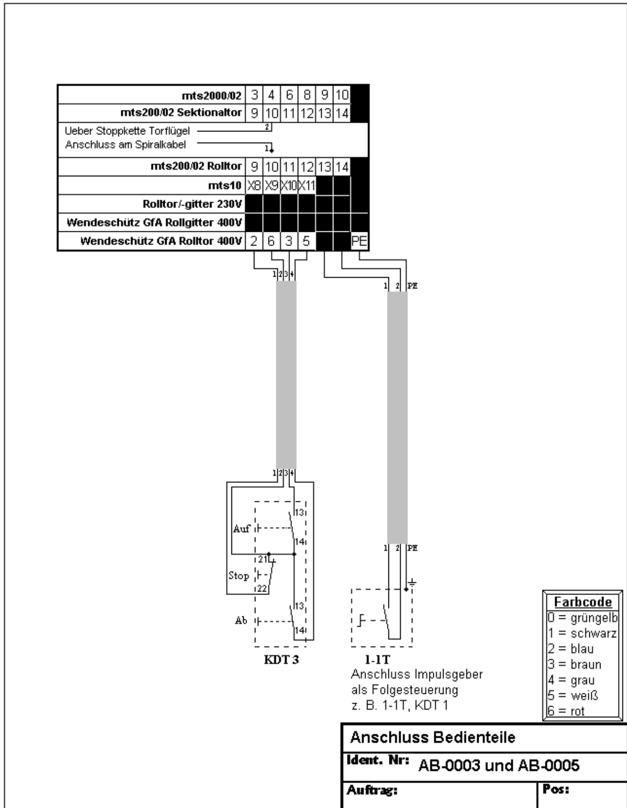
Abb. 11: Impulsgeber
