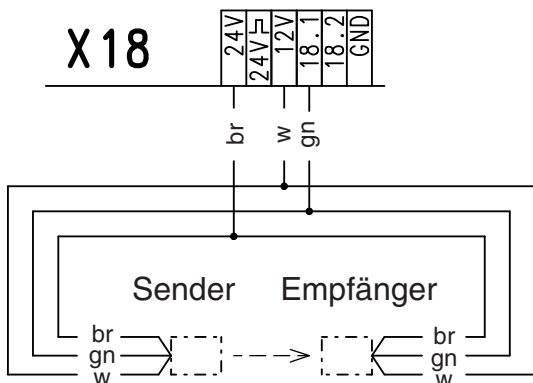
Rayctor Lichtschranke oder Optische Schaltleiste als Einzugssicherung einfach
