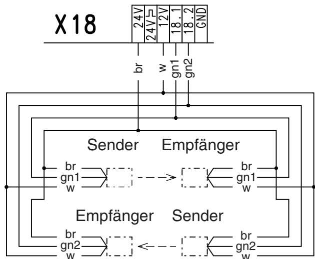
Rayctor Lichtschranke oder Optische Schaltleiste als Einzugssicherung zweifach
