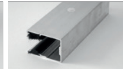
Laufschiene mit 2er-Bohrung und Abdeckkappe, wahlweise
