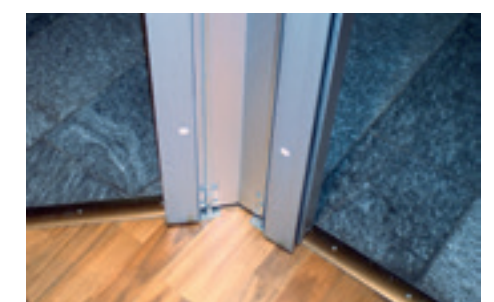
Detail: bei Bedarf verschiebbarer Mittelpfosten
