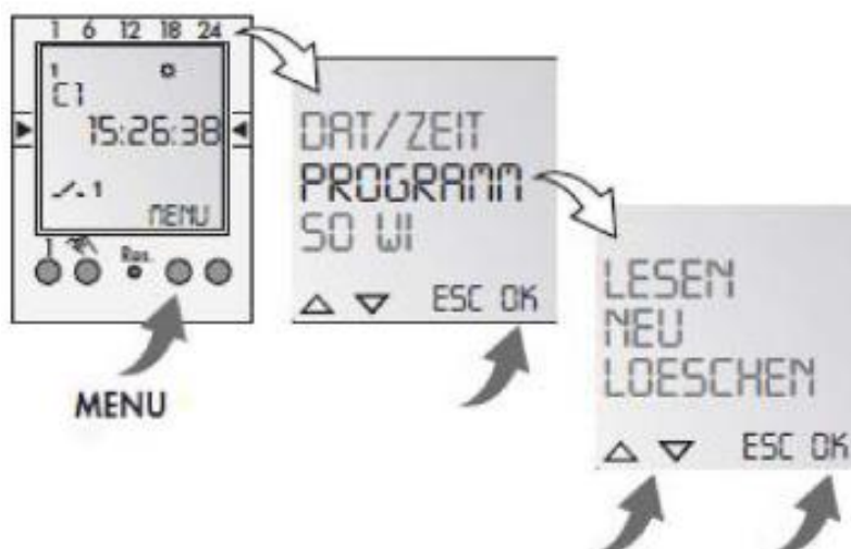
Abb. 8: Schaltuhr Erstinbetriebnahme – Wahl der Menüsprache
