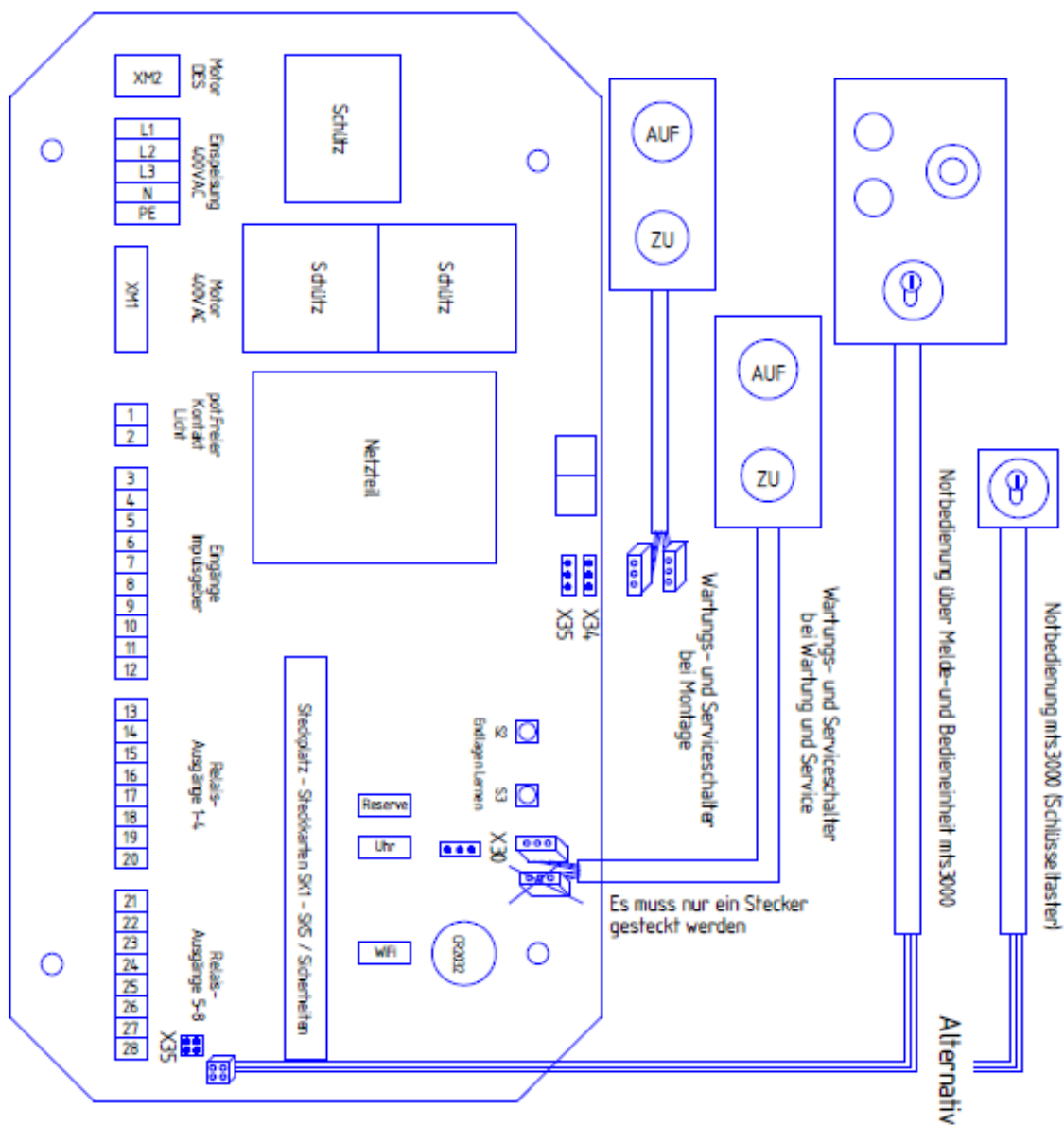
Abb. 7: Anschluss Handbedienungen
