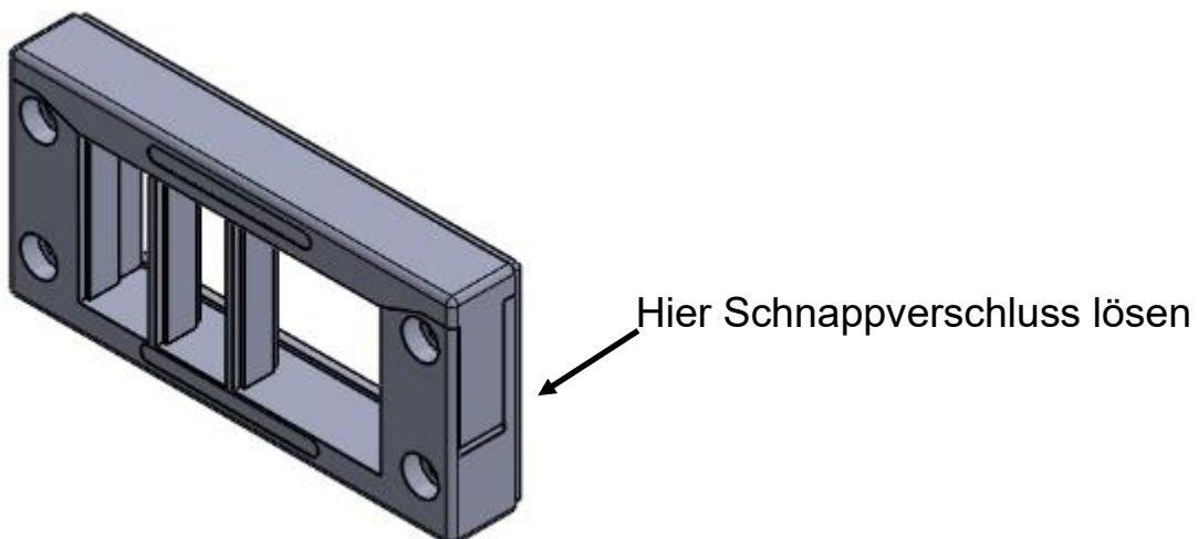
Abb. 2: Teilbare Kabeleinführungsleiste
