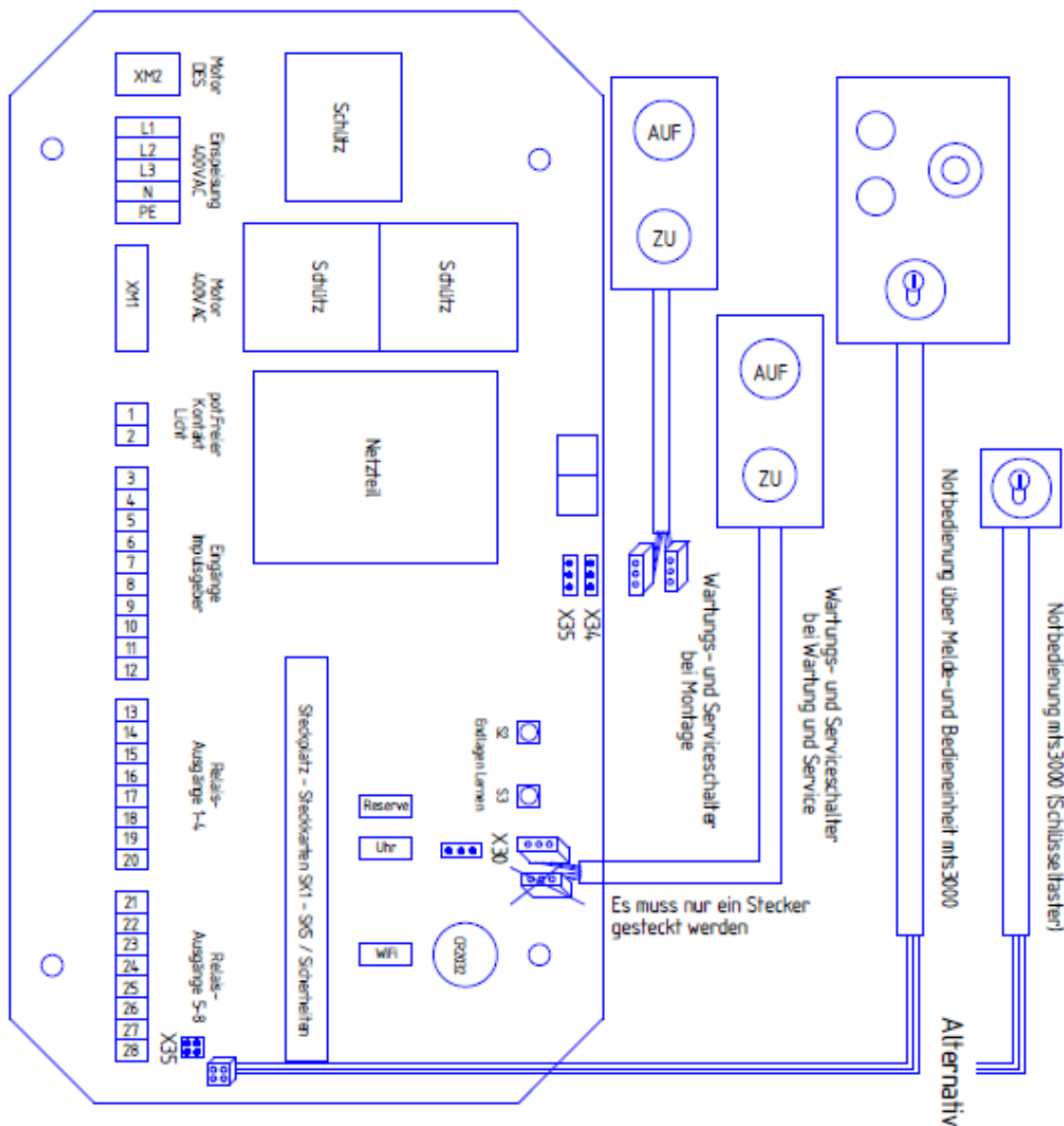
Abb. 7: Anschluss Handbedienungen
