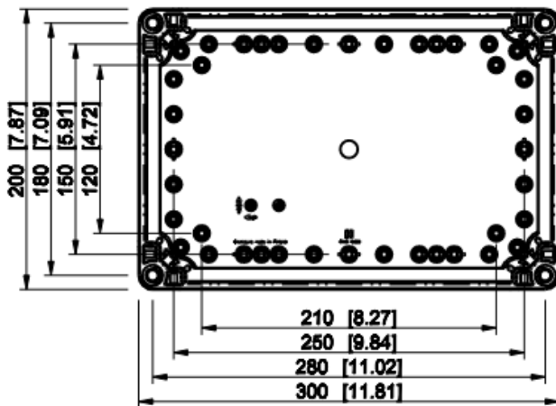
Abb. 3: Gehäuseabmessungen der Torsteuerung
